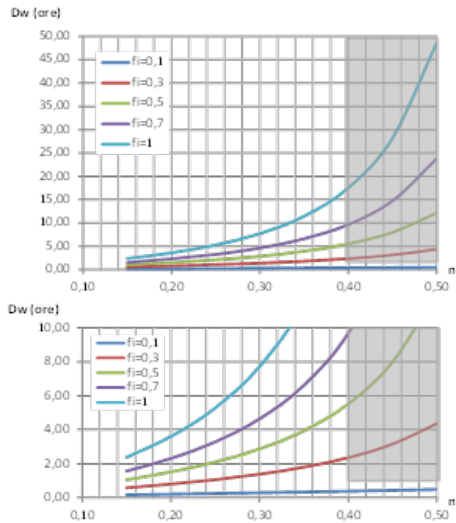
Figura 12 – Grafici della durata D_w (eq. 12») e del volume specifico critico di invaso w_c (eq. 13») in funzione di n , per \alpha=100 mm/ora e per u = 20 l/s per ettaro \alpha = 100 mm/ora n ; u = 20 l/s per ettaro
