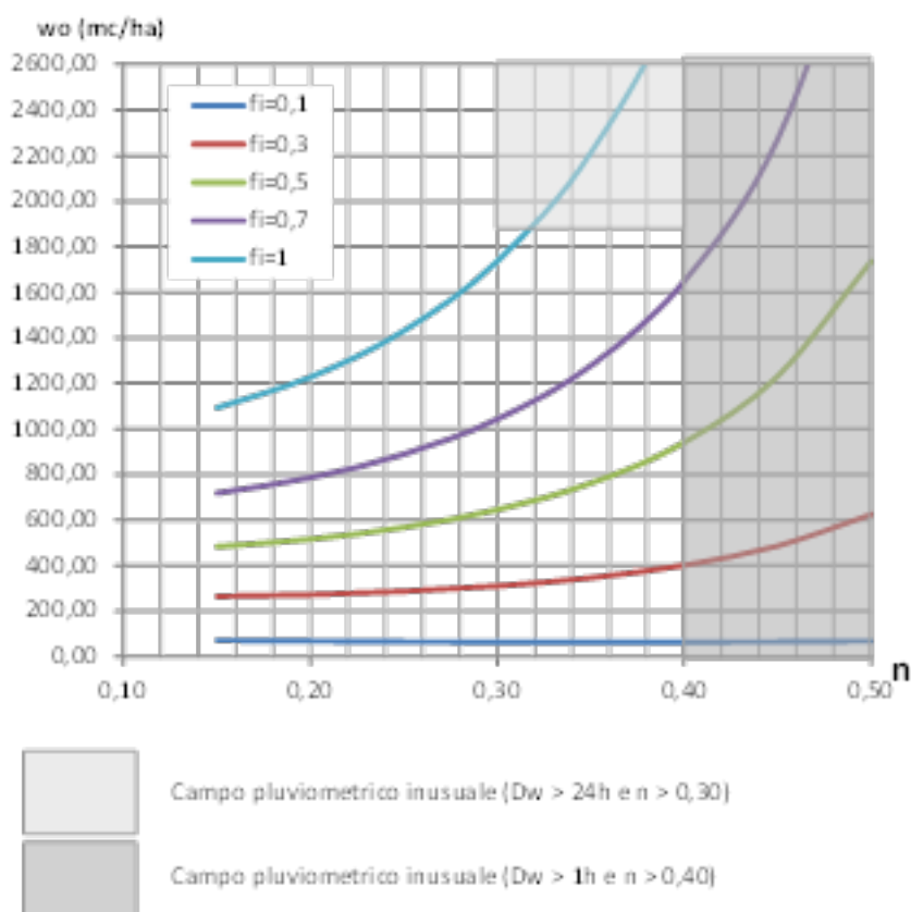
Figura 9 – Grafici della durata D_w (eq. 12») e del volume specifico critico di invaso w_o (eq. 13») in funzione di n , per \alpha=40 mm/ora e per u = 20 l/s per ettaro
