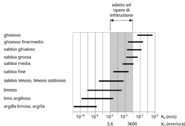
Figura 4: conducibilità idraulica per diverse classi tessiturali e condizioni ottimali di riferimento (modificato da DWA 2005)
