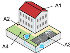
Figura 1: distribuzione delle superfici secondo l'ipotesi progettuale (A1: tetti e terrazze, A2: pavimentazioni semipermeabili, A3: pavimentazioni semipermeabili; A4: verde collettato).
